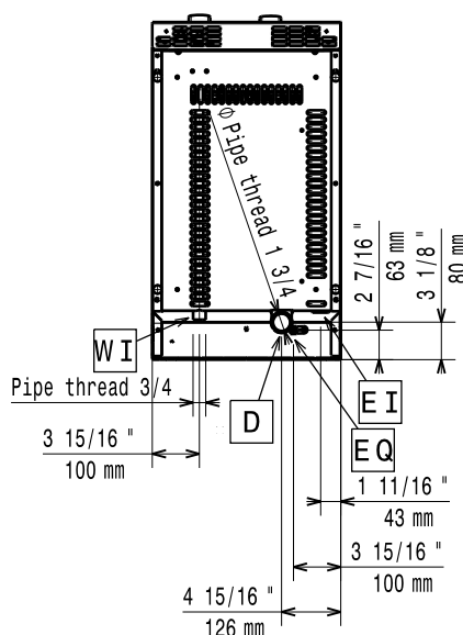
Boven aanzicht
